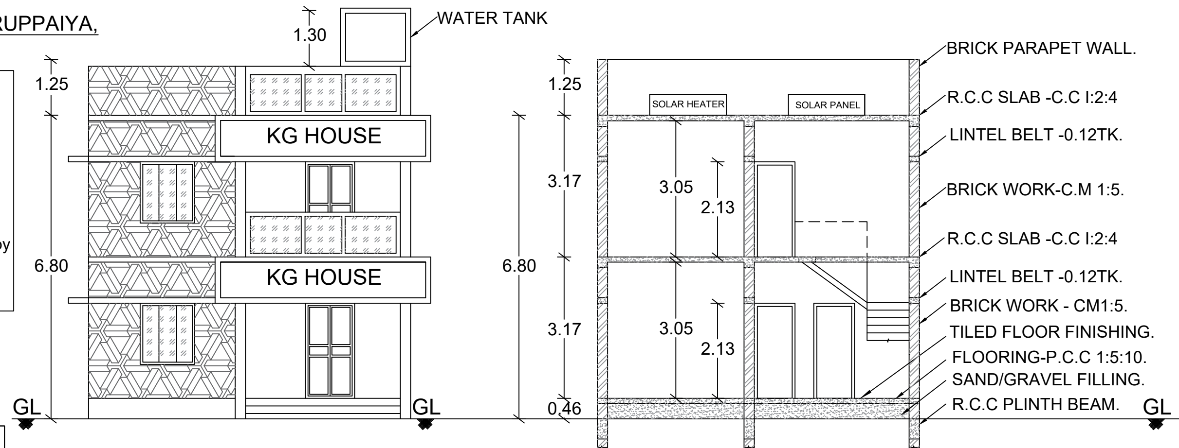
ELEVATION
