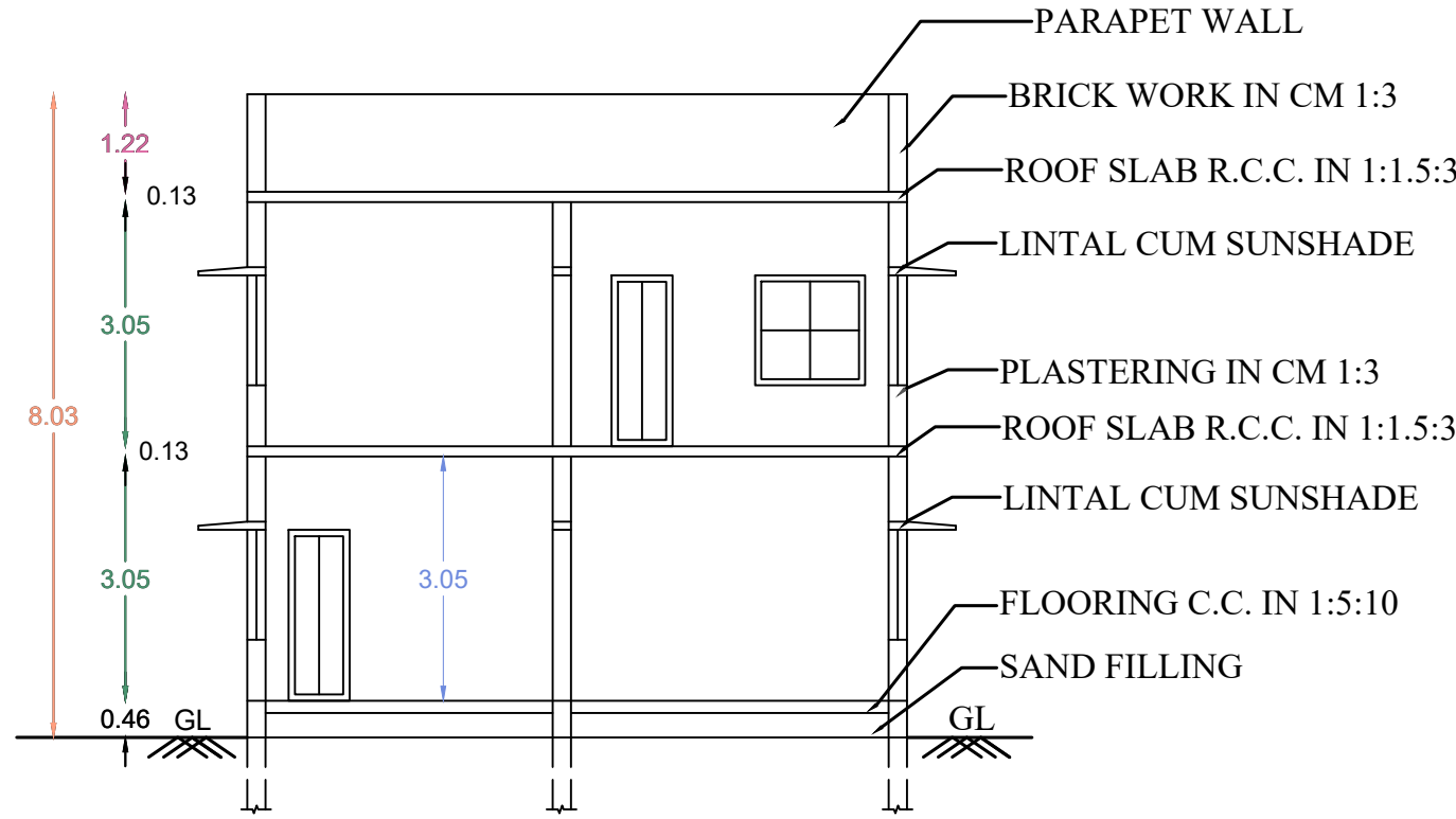
SECTION NO A-A
