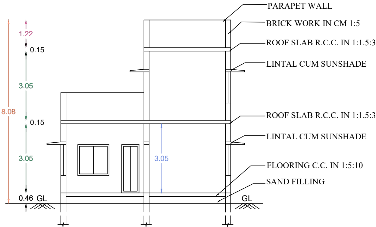
SECTION NO A-A
