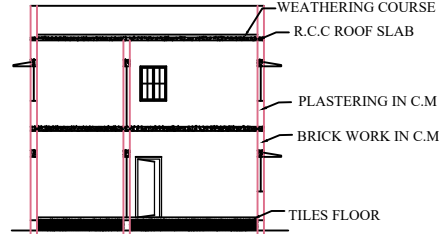
SECTION 'ab'
