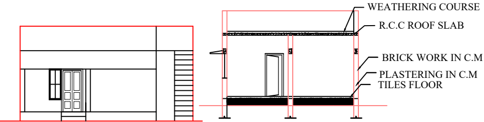
ELEVATION
