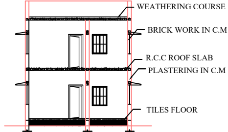
SECTION 'ab'
