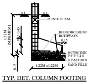
TYP. DET. COLUMN FOOTING
