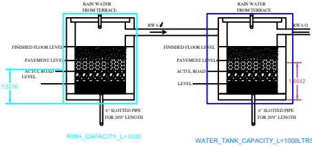
RWH_CAPACITY_L=1000
