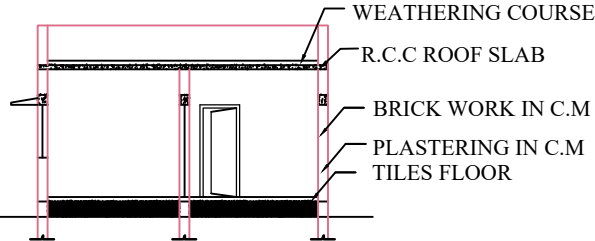
SECTION 'ab'
