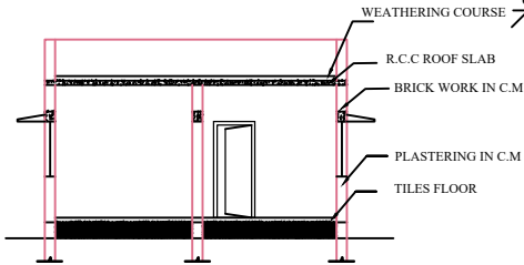
SECTION 'ab'
