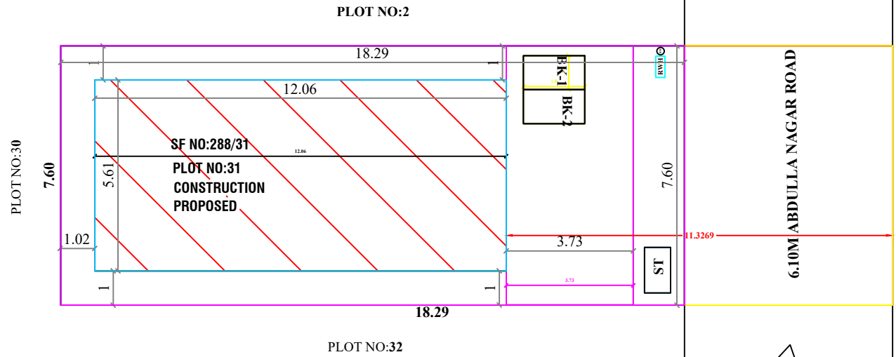
SITE-PLAN
