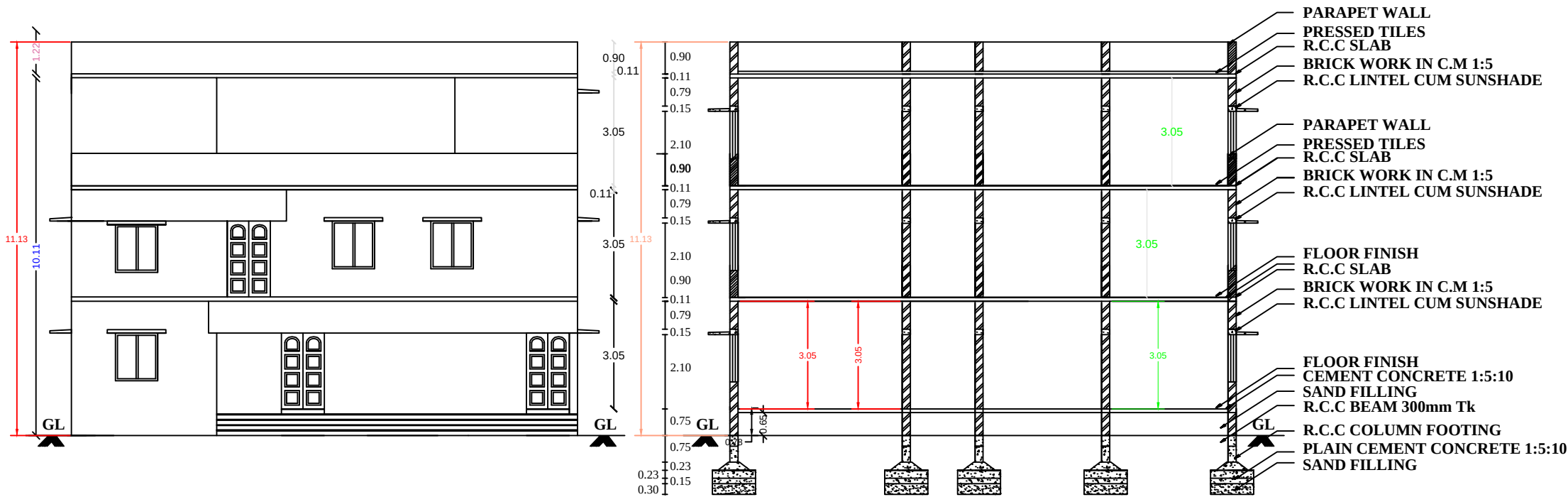
ELEVATION
