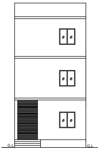
ELEVATION
