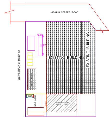
SITE PLAN SCALE: 1:250
