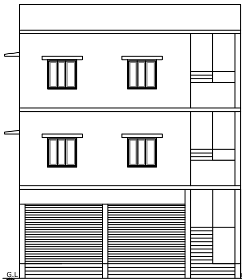
ELEVATION
