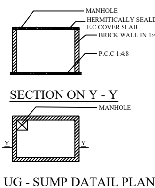
UG - SUMP DATAIL PLAN
