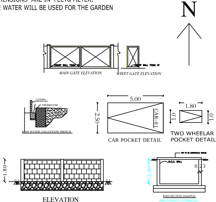
ELEVATION
