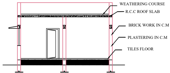
SECTION 'ab'
