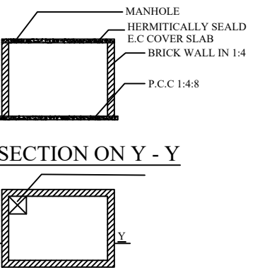
UG - SUMP DATAIL PLAN
