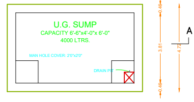
SUMP DETAIL SCALE: 1"=4'0"
