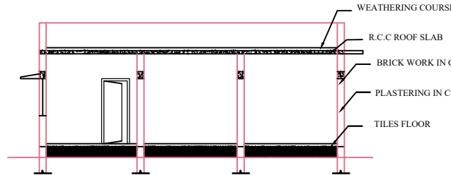
SECTION 'ab'
