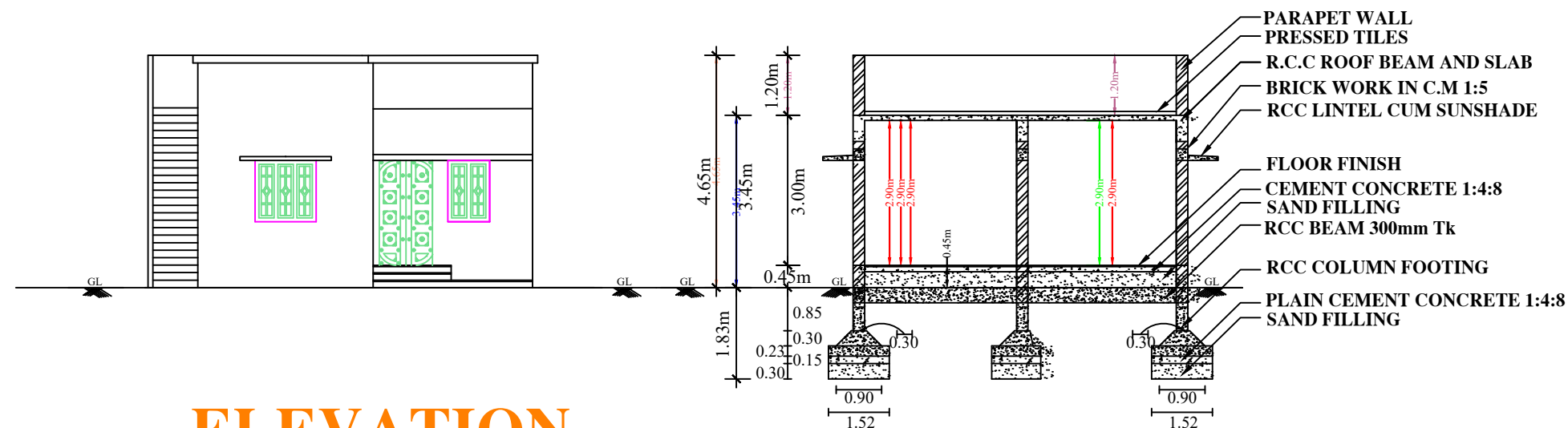
ELEVATION
