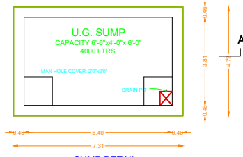
SUMP DETAIL SCALE: 1" = 2'-0"
