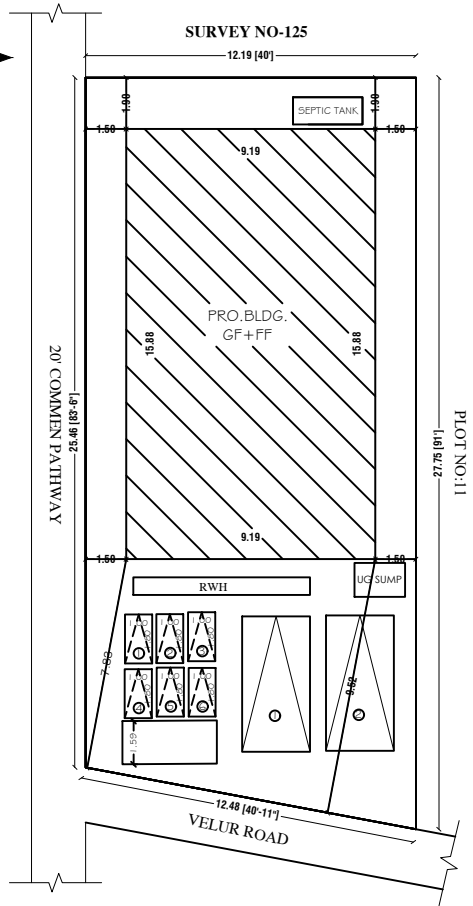
SITE PLAN 1:100
