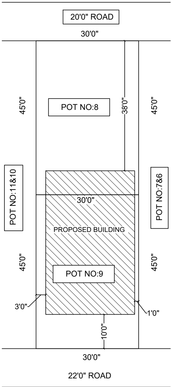
SITE PLAN NTS
