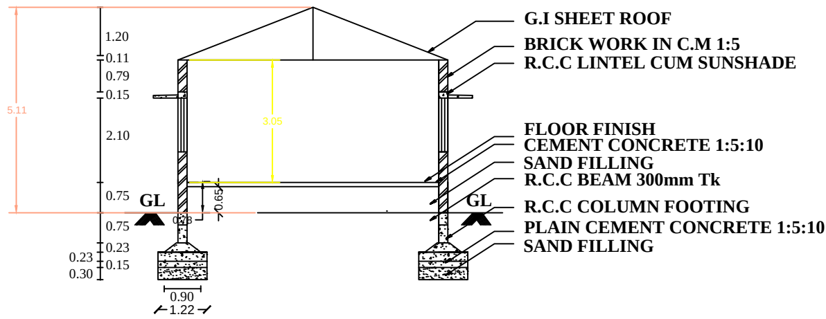
SECTION (A-A)
