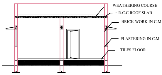
SECTION 'ab'
