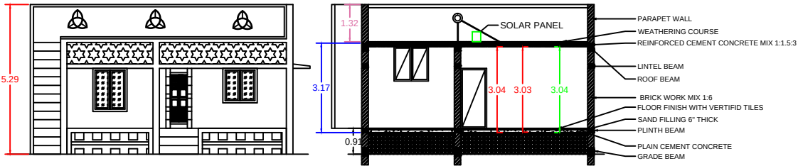
SECTION 'AB'
