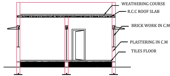
SECTION 'ab'
