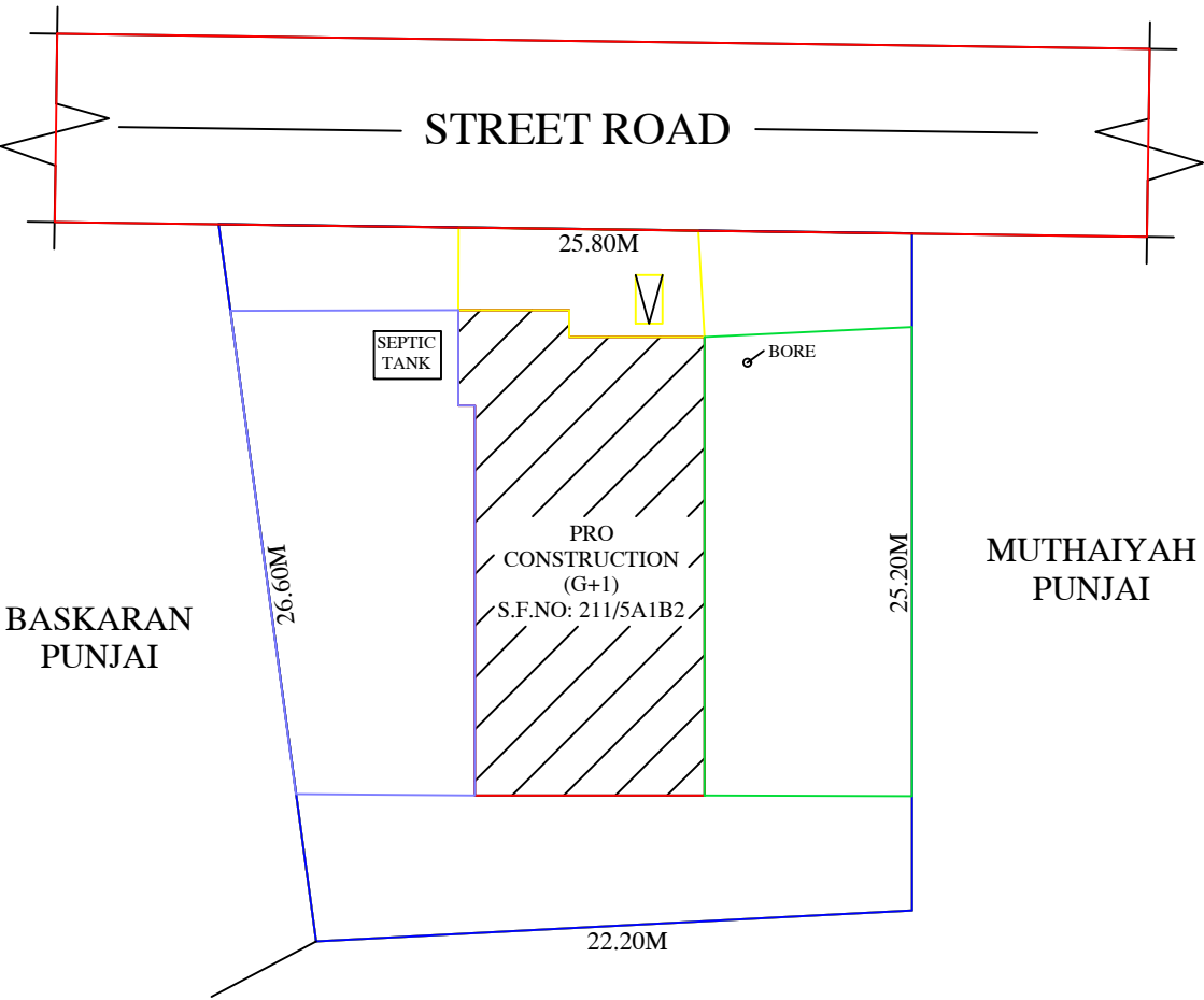
SITE PLAN:-
