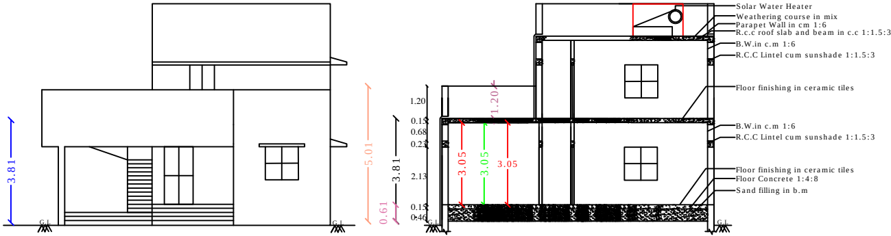
ELEVATION
