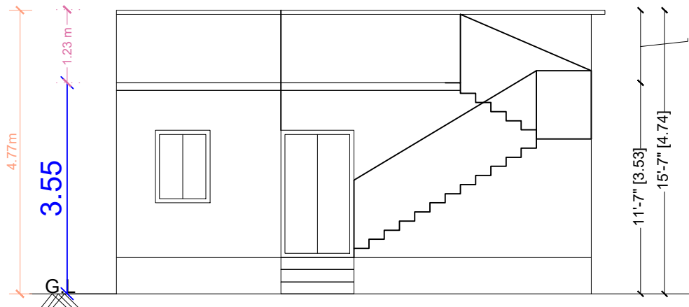
ELEVATION
