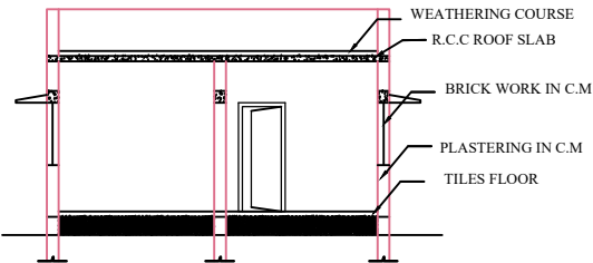
SECTION 'ab'
