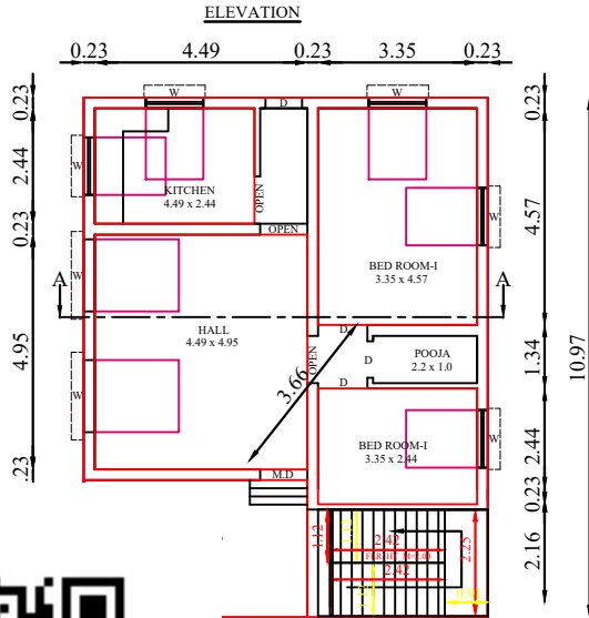
UND FLOOR PLAN SCALE 1: 100
