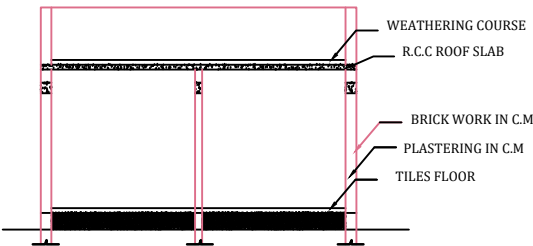
SECTION 'ab'
