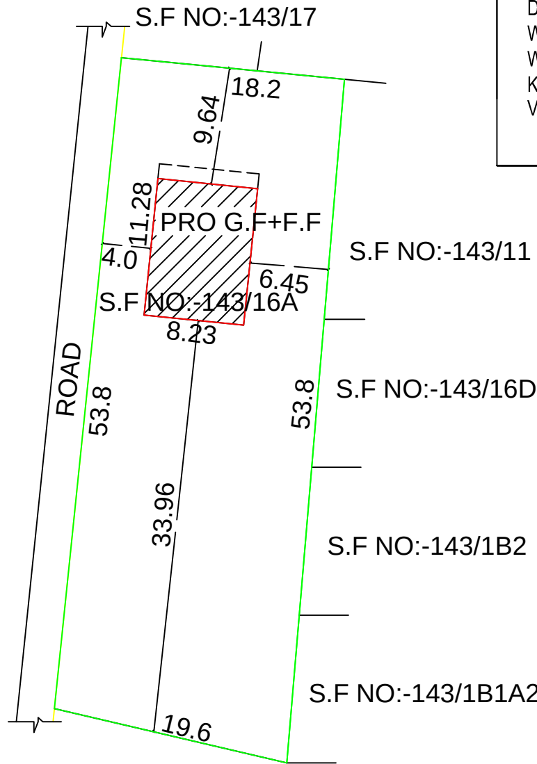
S.F NO:-143/13
