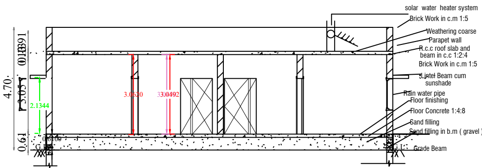
SECTION A-A
