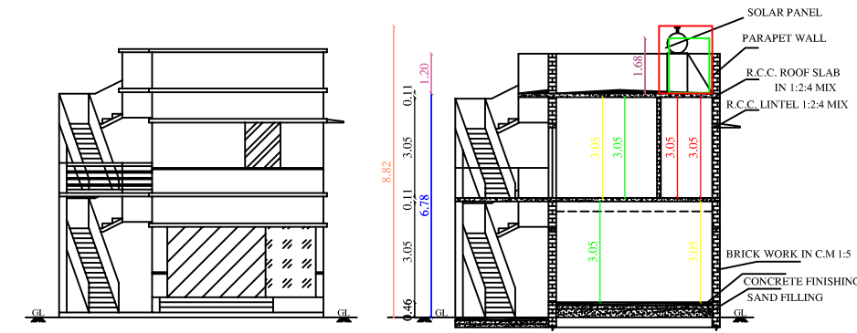
ELEVATION
