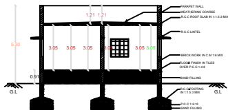
SECTION -AB
