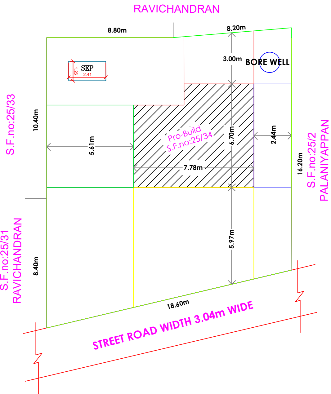
SITE PLAN-SCALE 1:100
