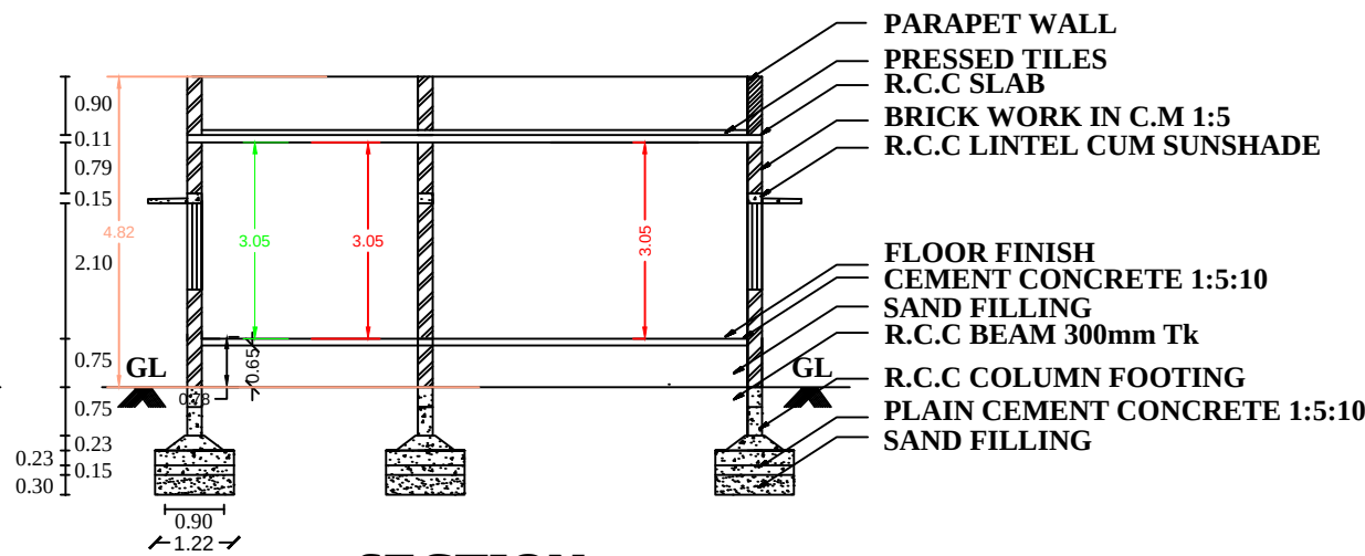
SECTION (A-A)
