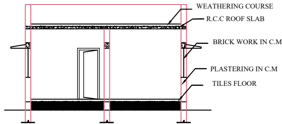
SECTION 'ab'
