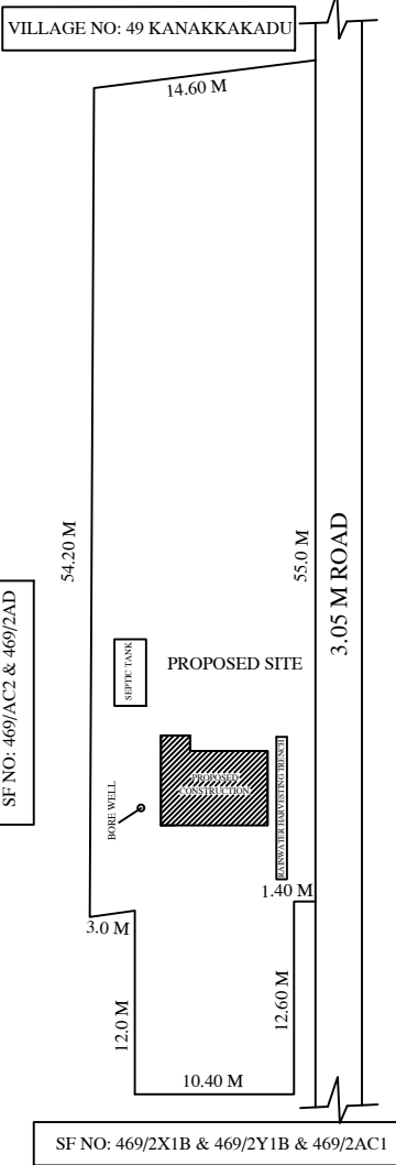
SITE PLAN (scale -1:200)
