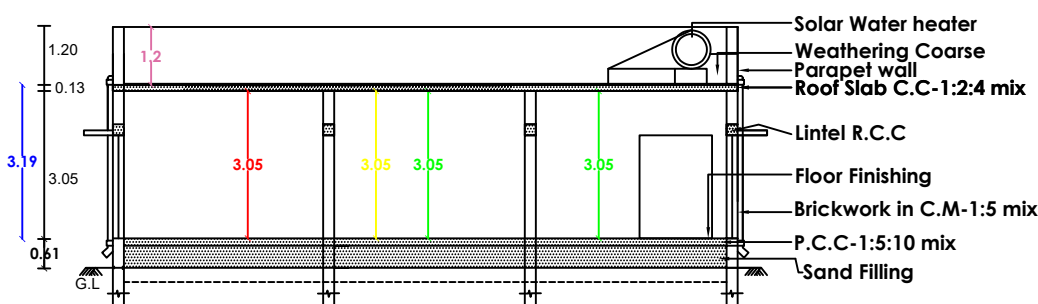
SECTION 'AB'
