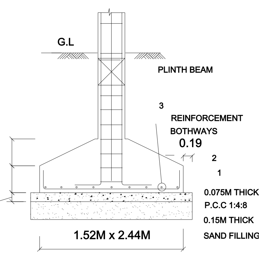
TYP. DET. COLUMN FOOTING
