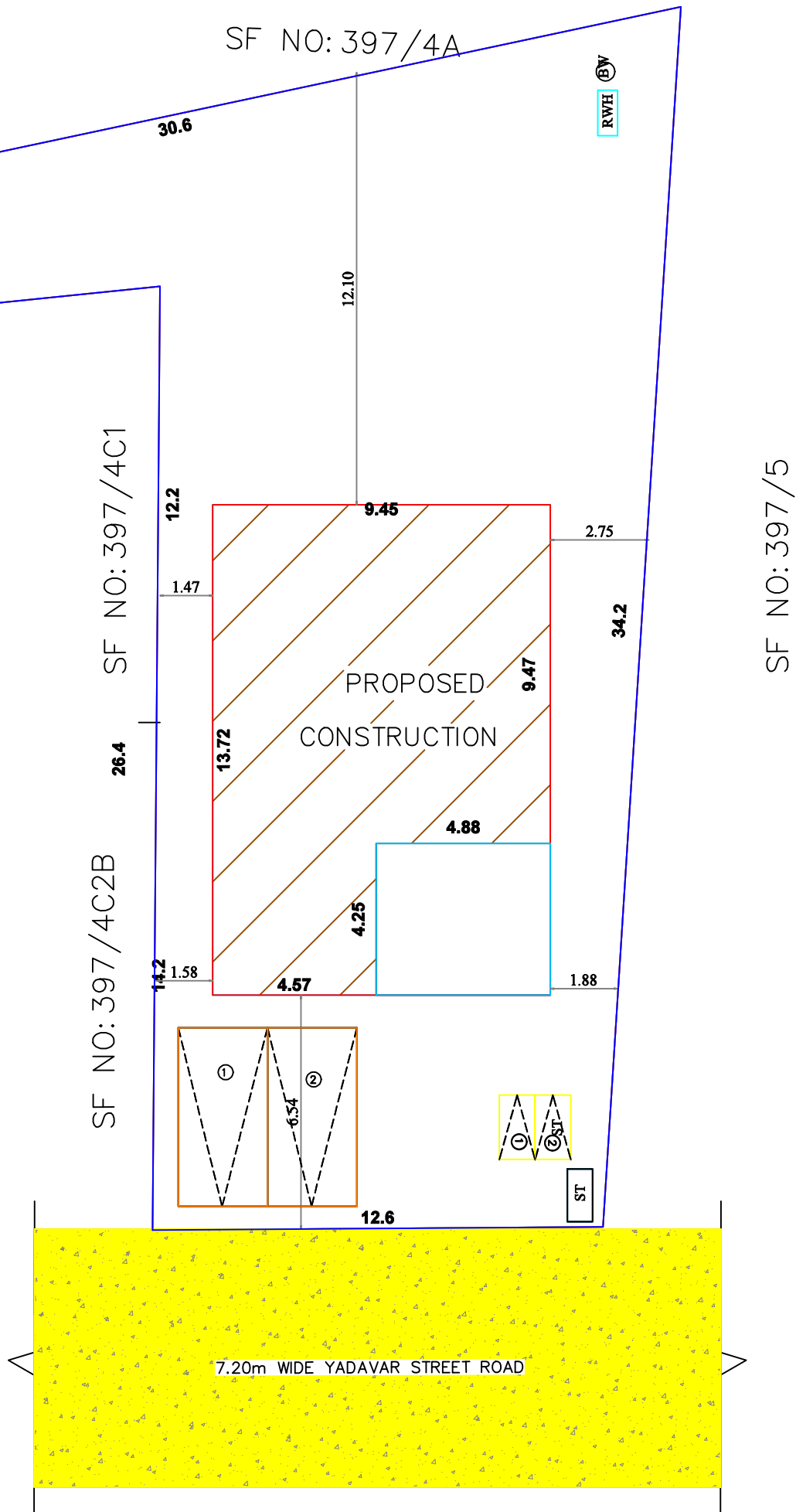
SITE-PLAN
