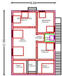
G. FLOOR PLAN
