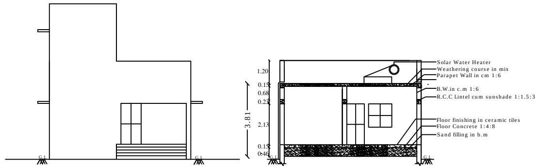
ELEVATION
