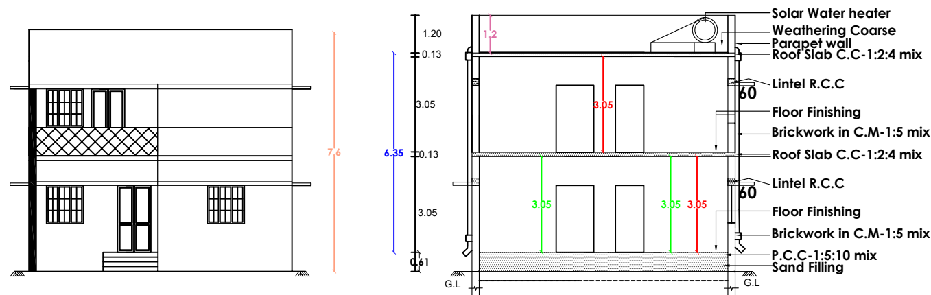
ELEVATION
