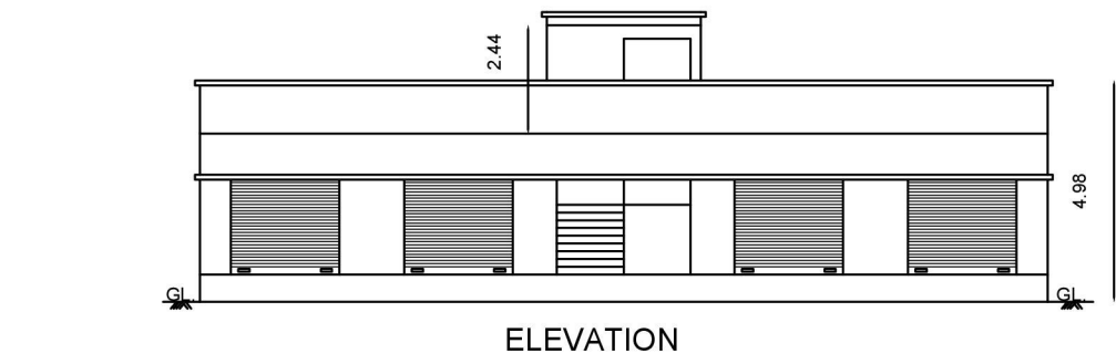
ELEVATION
