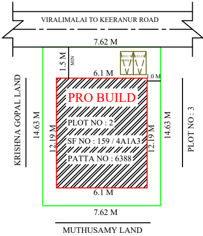
SITE PLAN SCALE 1:400
